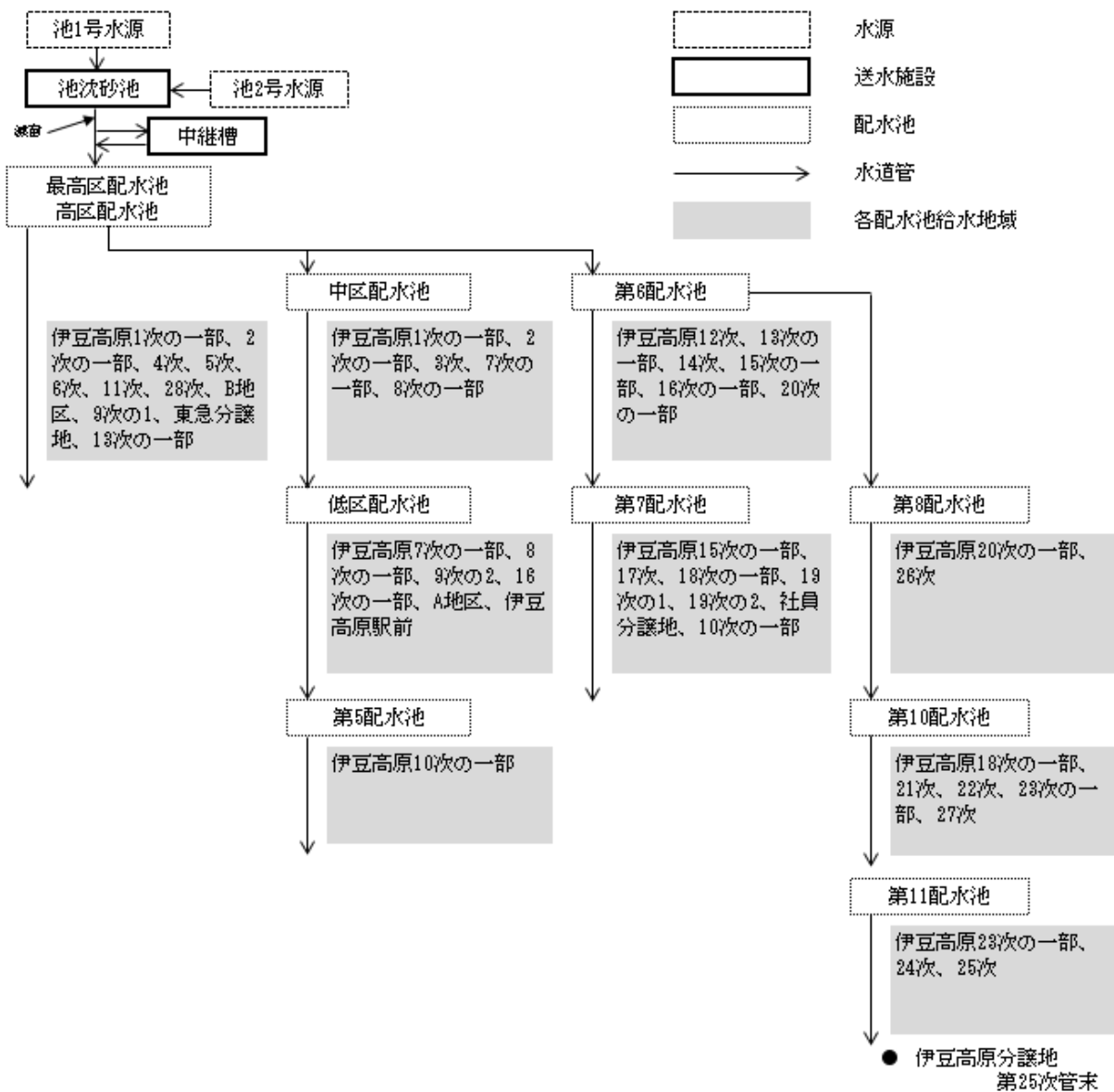
伊豆高原水道事業給水系統図
